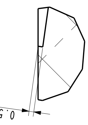
DETAIL B ECHELLE 4:1
